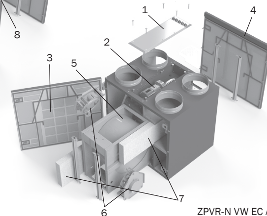
ZPVR-N VW EC A
